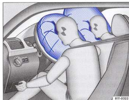
Fig. 23 Imagine de referință: Airbag frontal declanșat văzut din lateral.
