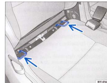
Fig. 40 Inelele de ancorare a scaunelor pentru copii cu sistem ISOFIX în ramele scaunelor laterale din al doilea rând de scaune.
