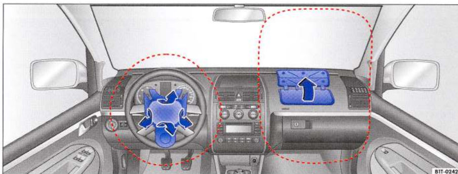
Fig. 28 Zona de acțiune și capacele airbag-urilor la declanșarea airbag-urilor frontale.
