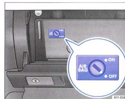
Fig. 33 Torpedoul de pe partea pasagerului din dreapta: Întrerupător cu cheie pentru dezactivarea și activarea airbag-ului frontal al pasagerului din dreapta.
